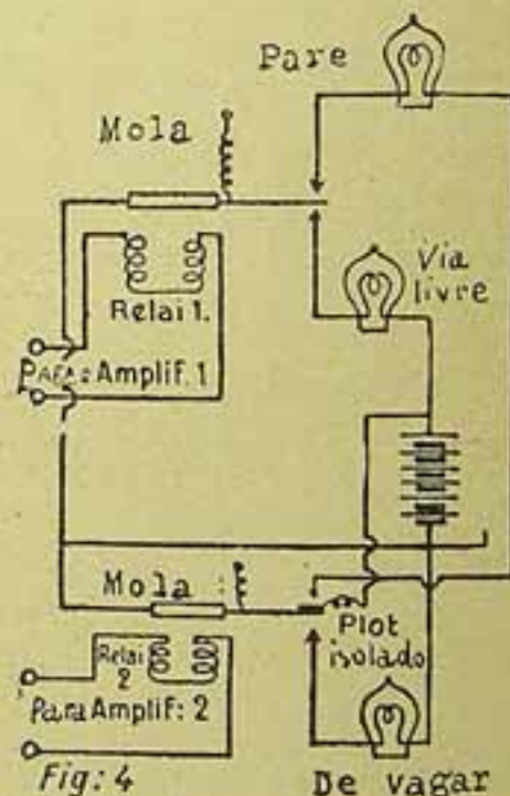
(Fig. 4) — Funcionamento dos relais
