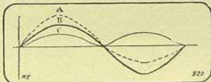
(Fig. 2) — ONDAS APPLICADAS AO APARELHO RECEPTOR. — A, onda complexa representando a corrente filamento placa das lâmpadas montadas em push-pull; B, onda fundamental; C, onda harmonica
