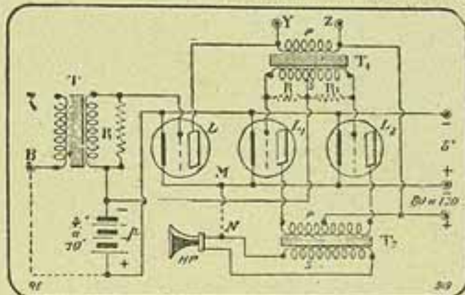
(Fig. 1) — MONTAGEM PUSH-PULL COLLOCADA EM SEGUIDA A UM DETECTOR DE GALENA OU DE LÂMPADAS, ALIMENTADO EM CORRENTE CONTINUA. — A, B, bornes do transformador de entrada T; R, R1, resistencias em derivação; p, pilha para tensão de grade; L, L1, lâmpadas; T1, T2, transformadores para montagem push-pull; M, N, curto-circuito; H, P, auto-falante; Y, Z, bornes de circuito primario de vai vem
