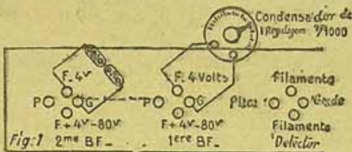
(Fig. 1) — Montagem externa
