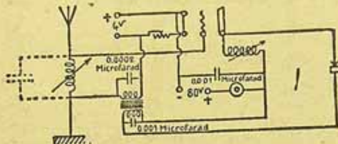
(Fig. 1) — Schema da montagem
