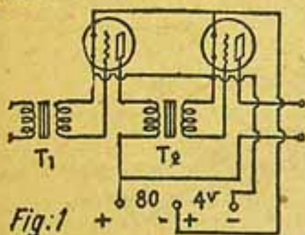
(Fig. 1) — Schema de principio
