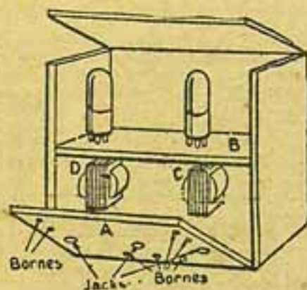
(Fig. 3) — Disposição dos aparelhos: A, painel da frente; B, painel das válvulas, em ebonite; C, transformador de ligação, T2; D, transformador de entrada T1
