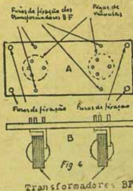
(Fig. 4) — A, vista da planta baixa; B, vista do plateau d-elevação do aparelho
