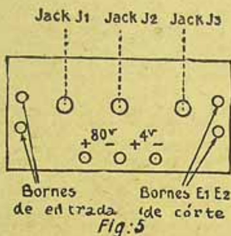
(Fig 5) — Disposição dos Jacks
