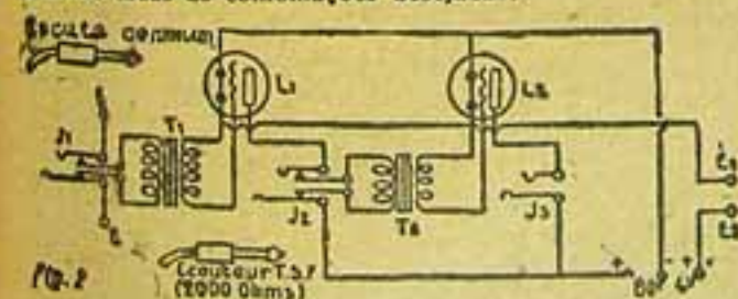
(Fig. 2) — Schema da montaggio
