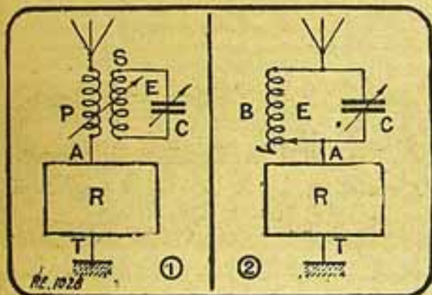
FIGURA 1 — MONTAGEM DE UM CIRCUITO ELIMINADOR NA ANTENNA DE RECEPÇÃO. — I — Montagem directa: A, berne da antenna; T, berne da terra do receptor R; P, bobina de acoplamento intercalada na antenna; S, bobina de eliminador; C, condensador. — II — Montagem directa: B, bobina do eliminador; C, condensador.
