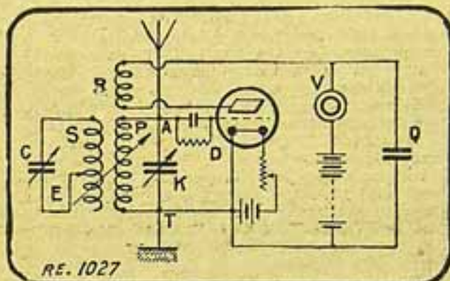
FIGURA 2 — MONTAGEM DE CIRCUITO EM ELIMINADOR, ACOPLADO COM UM RECEPTOR MONTADO DIRECTO. — E, eliminador; S, bobina do eliminador; C, condensador de regulagem do eliminador; R, reacção; A, antenna; T, terra. P, K., bobina e condensador de regulagem da estação; D, condensador shuntado de detecção.
