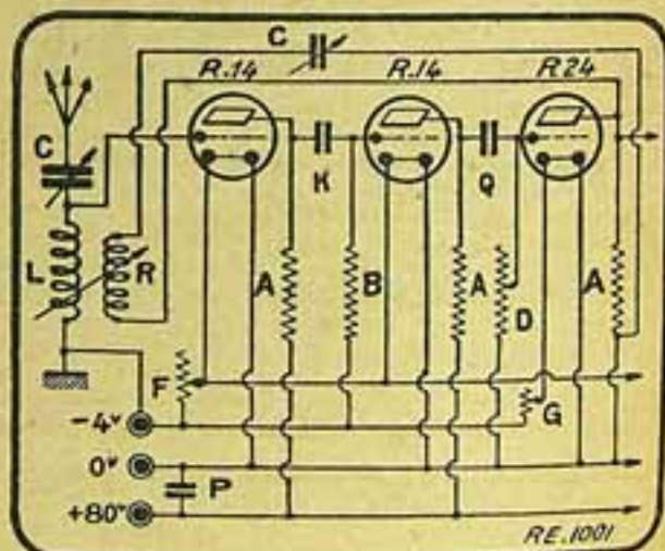
Fig. — II — Amplificador detector de resistencia comportando duas classes de amplificação de alta frequência e uma lampada detectora. — Mesma legenda que para a Fig. 1, com a unica differença de que o condensador fixo de conexão K é de 0,0005 de micropharadi. Circuito de reacção sobre a valvula detectora.
