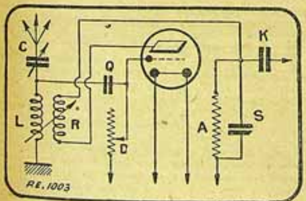
Fig. IV — Novo dispositivo de reacção. — Mesma legenda que para a Fig. 1. — S, condensador fixo de 5,005 microphardi evitando a passagem do corrente de alta frequência através da resistencia da placa A.
