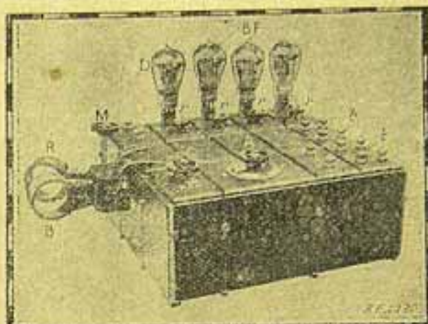
Fig. 5 — V — Realização de um amplificador detector de resistencia. — A, condensador de afinação; B, bobina de accordo (afinação); M, maneta de reacção; C, commutador ondas curtas; ondas longas; R, rheostatos de aquecimento; D, válvula detectora; D. F., válvulas amplificadoras; D, bornes; R, reacção acoplada pela bobina de afinação.
