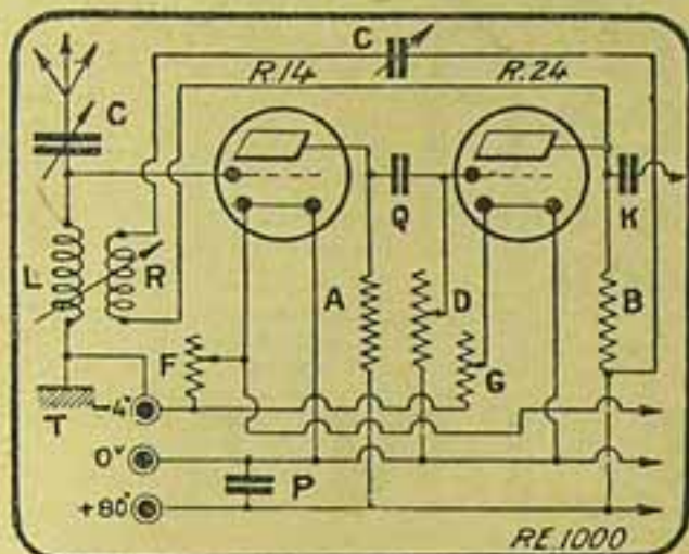
Fig. — I — Amplificador detector de resistencia comportando uma instalação de amplificação de alta frequência e uma valvula detectora. — C, condensadores variaveis de ar, de 0,0005 a 0,001 micropharadi; L, bobina de accordo; T, terra; R, bobina de reacção; Q, condensador de detecção (0,0002 micropharadi); K, condensador fixo de conexão de 0,006 micropharadi; A, resistencia de 200.000 ohms; P, resistencia de 15 megohms; F, rheostato de aquecimento das valvulas amplificadoras; G, rheostato de aquecimento da valvula detectora; D, resistencia variavel de 0,5 a 15 megohms; P, condensador fixo de 2 micropharadis.
