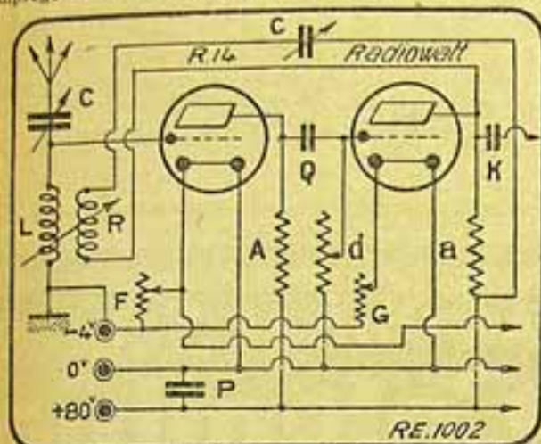
Fig. 111 — Amplificador detector de resistencia comportando uma instalação de alta frequência seguida de uma válvula detectora radiowatt. — Mesma legenda que para a Fig. 1, com as modificações seguintes: D, resistencia variável de 50.000 ohms ou menos; A, resistencia fixa de 15.000 mais ou menos; G, rheostato continua para a válvula de consumo normal.
