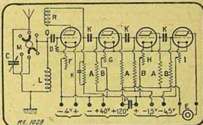
Fig. VI — Schema de amplificador detector de resistencia representado pela Fig. 5. — C, condensador variavel; L, bobina de afinação; R, reacção; Q, condensador de detecção de 0,0002 microphardi; D, resistencia fixa de dois megohms; F, G, H, I, rheostato de encandecimento; K, condensador fixo de 0,005 de microphardi; A, resistencia de 200.000 ohms; B, resistencia de 15 megohms; P, condensador fixo de dois microphardi; E, auto fallante; M, commutador.
