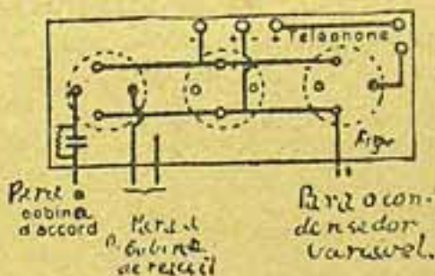
Fig. 3 — Ligações do painel de lampadas
