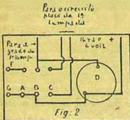
Fig. 2 — A suporte do self de antenna; B, suporte fixo do self de accôrdo; C, suporte do self de reacção; D, condensador variavel; F, G, antenas e terra
