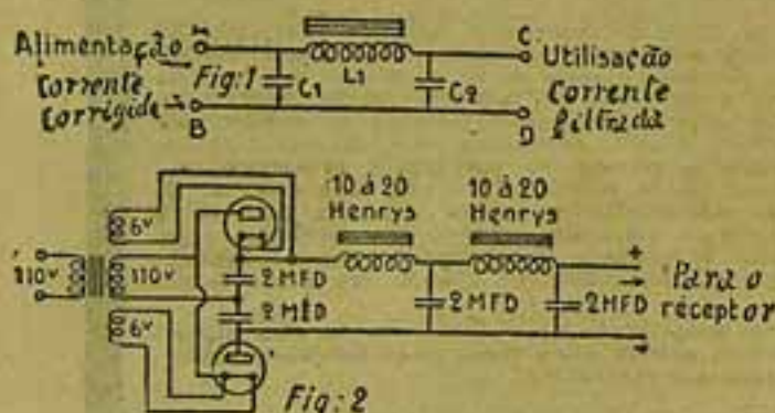
Fig. 1 — Schema de principio
