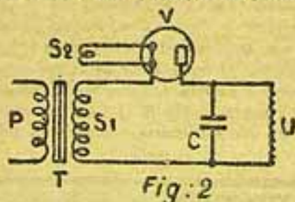
(Fig. 2) — Correção de um meio-periodo alternativo por uma valvula e um condensador. Designação no Commercio (T, transformador... 110/110/6 V, C, condensador de 2 microfarad)
