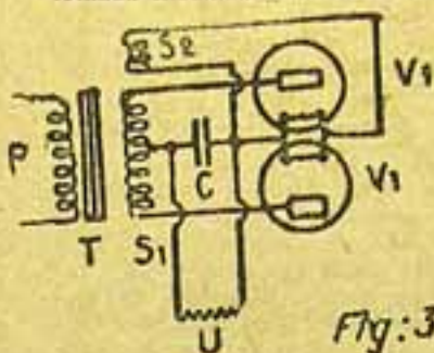
(Fig. 3) — Correção de um periodo de corrente alternativa por duas valvulas e um condensador. (T, transformador 110/110/110/6 V. C., condensador de 2 microfarad)
