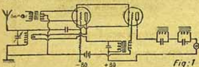
(Fig. 1) — Alimentação de uma detectora e de uma amplificadora BF pela corrente alternativa do sector
