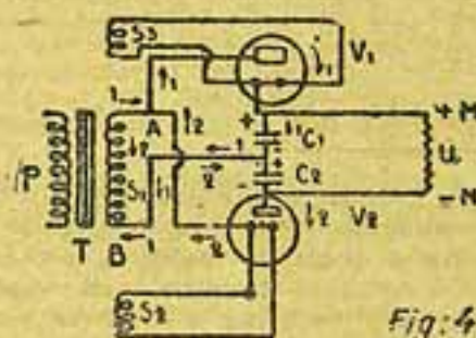
(Fig. 4) — Correção de um periodo de corrente alternativa por duas valvulas e dois condensadores. (T, transformador 110/65/6/6 V. C1 e C2 condensadores de 2 microfarad)
