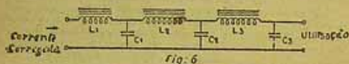
(Fig. 6) — Dispositivo de filtros
