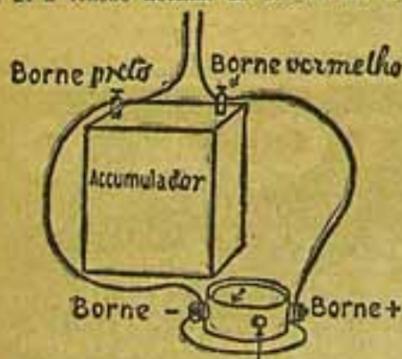
(Fig. 2) — Medida da tensão dos acumuladores
