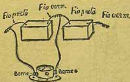
(Fig. 3) — Medida da tensão das pilhas
