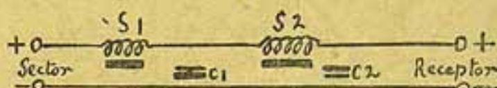
2 Estagios de filtro
