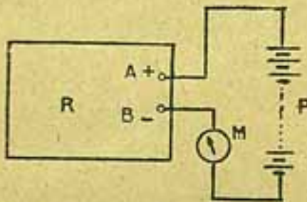
Fig. 3 — R receptor; A e B bones + e - 80 v ; M milliamperemetro; P bateria de pilhas de placa
