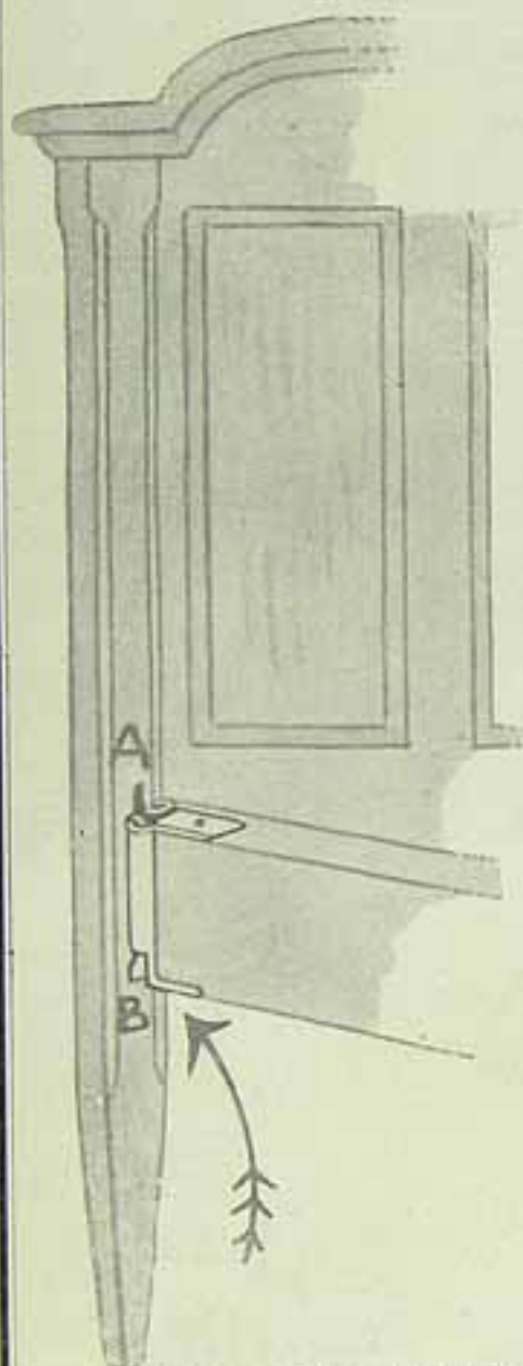
A parte A-B fica invisivel pelo encaixe da peça C.
