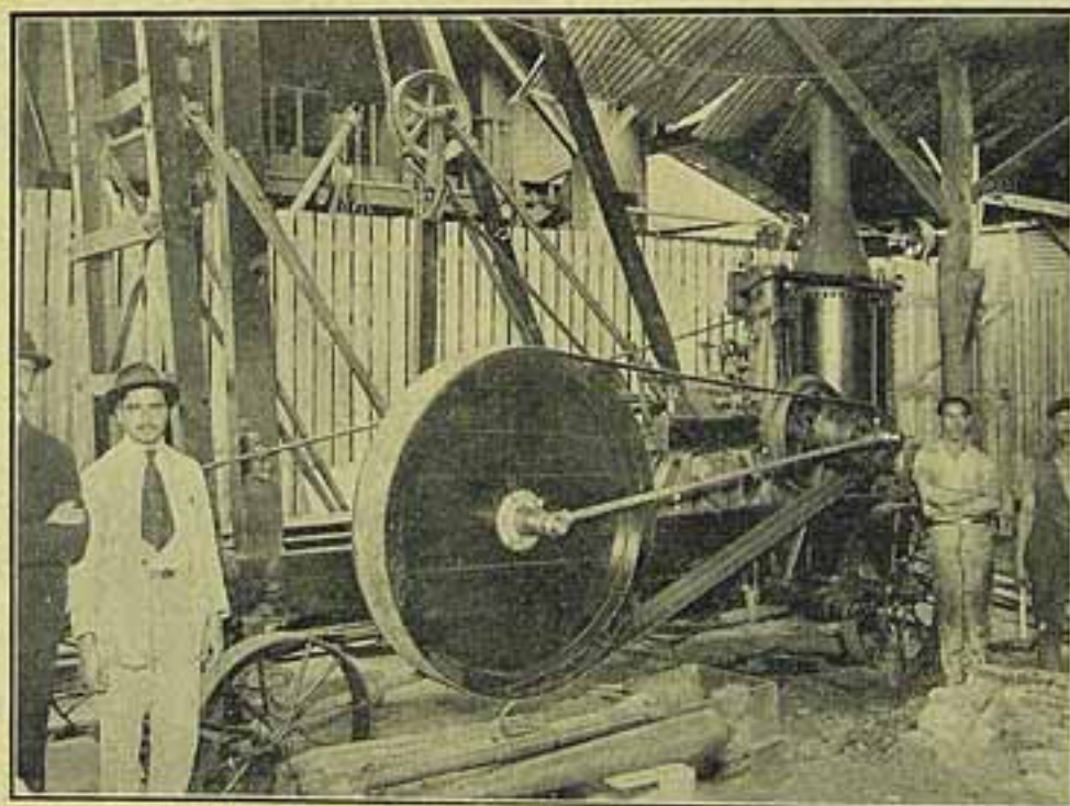
Vista lateral
