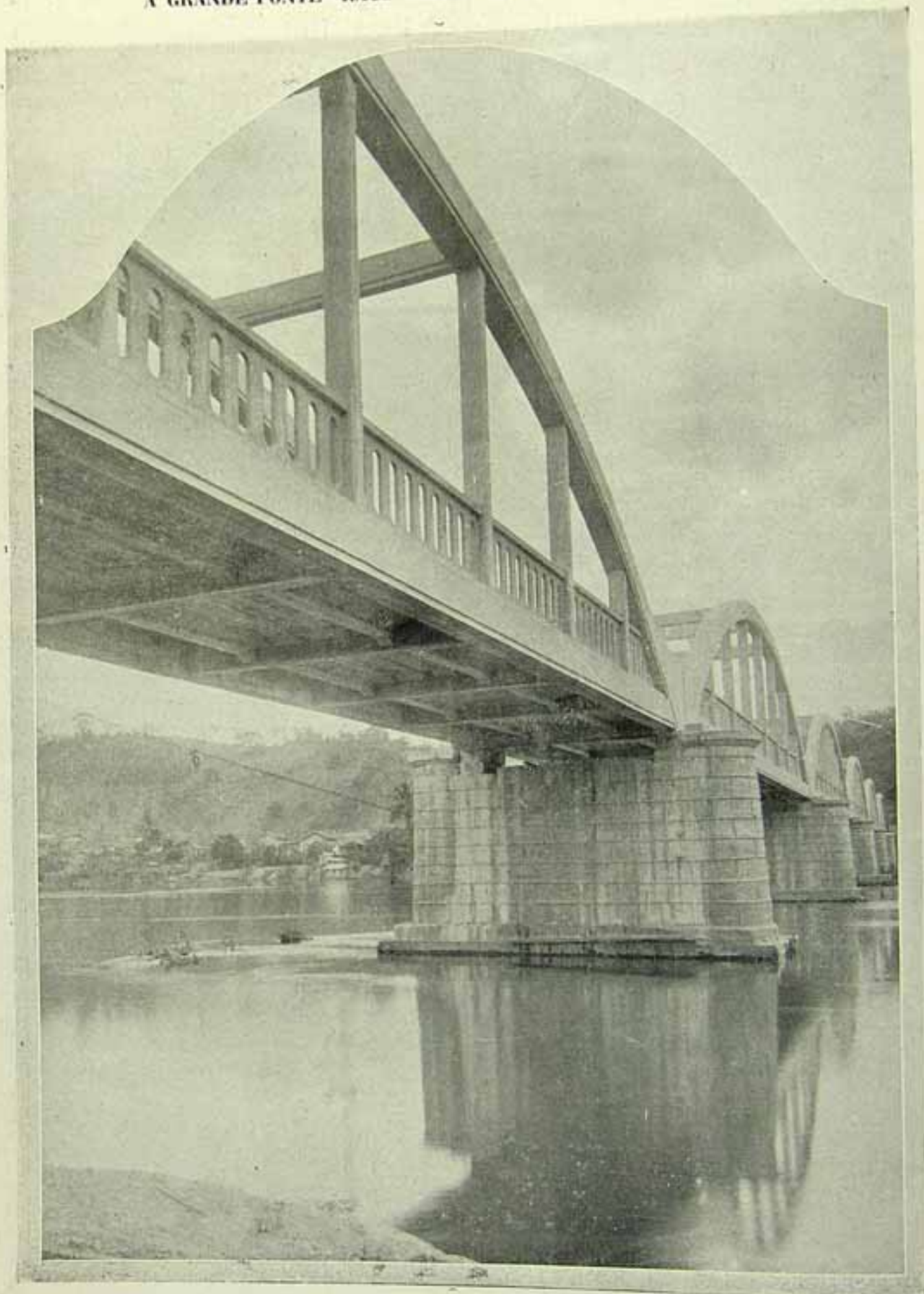
Um aspecto da ponte "Raul Veiga", para mostrar principalmente a solidez dos pilares e do leito da mesma ponte
