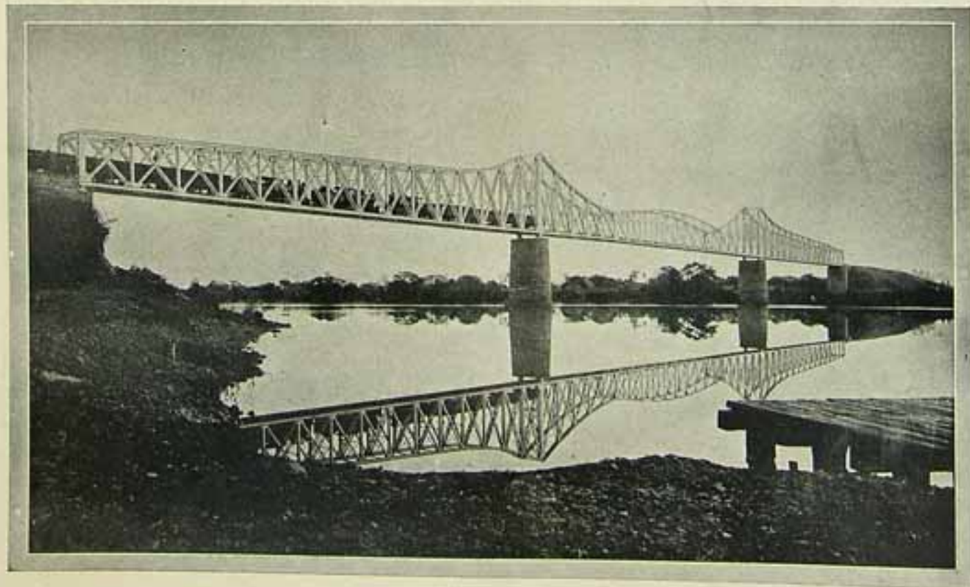
A nova e importante ponte sobre o rio Taquary—Rio Grande do Sul. Photographia tirada no dia da experiencia, ao lado da Volta do Barreto.
