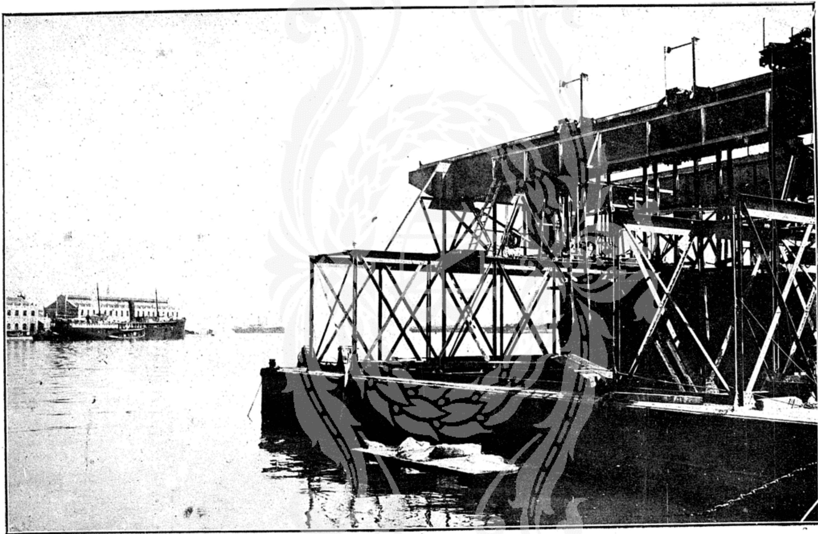
O PRIMEIRO PYLONE CONSTRUÍDO ACIMA DA MARÉ MÍNIMA — O CÃES DE ATRACAÇÃO, QUANDO PROMPTO, TERÁ UMA EXTENSÃO DE 3 KILOMETROS.
