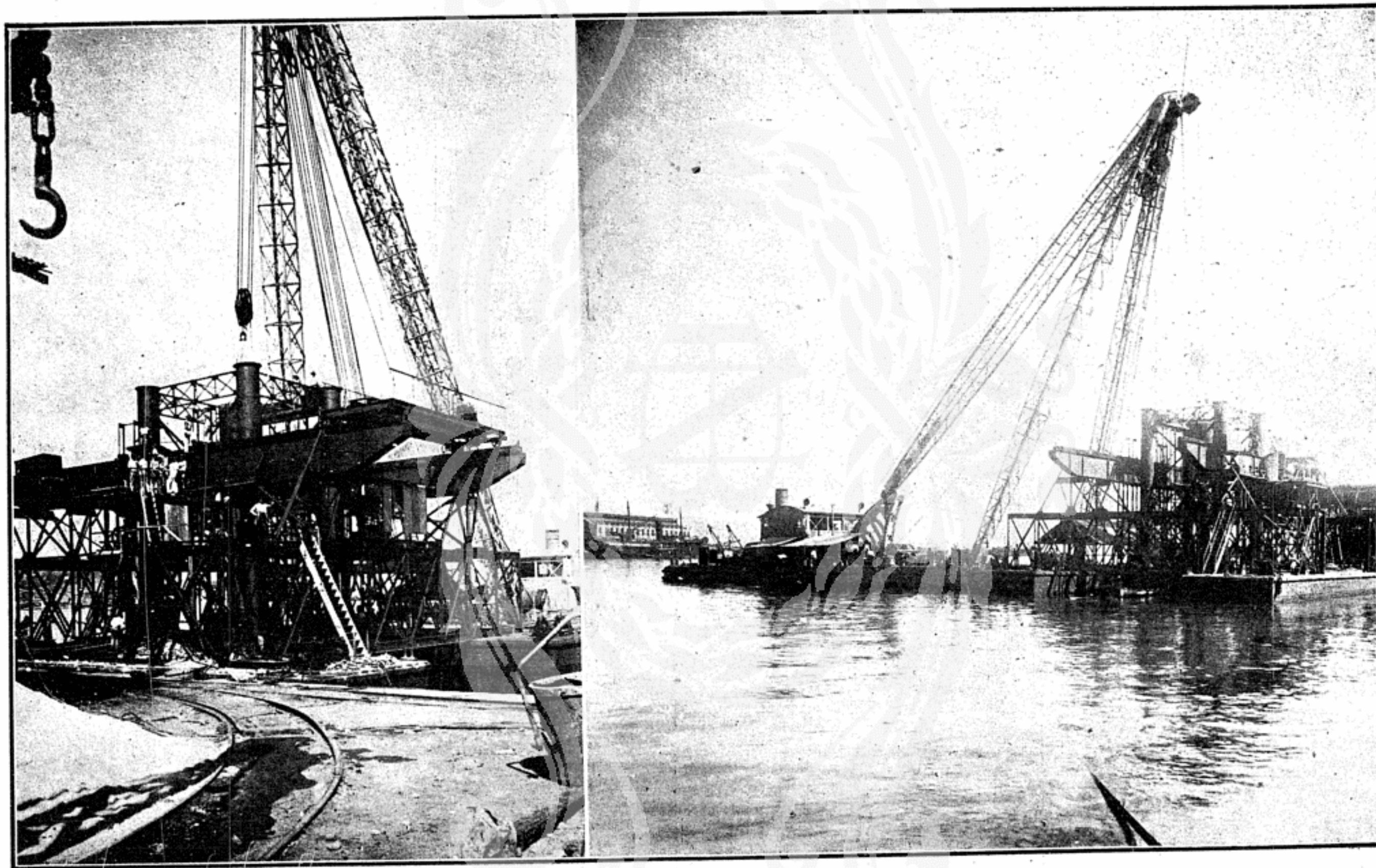
1 E 2 — COLLOCAÇÃO DA CAMPANULA NO CAIXÃO DE AR COMPRIMIDO NUMERO 2 PELA CABREA MARECHAL DE FERRO.
