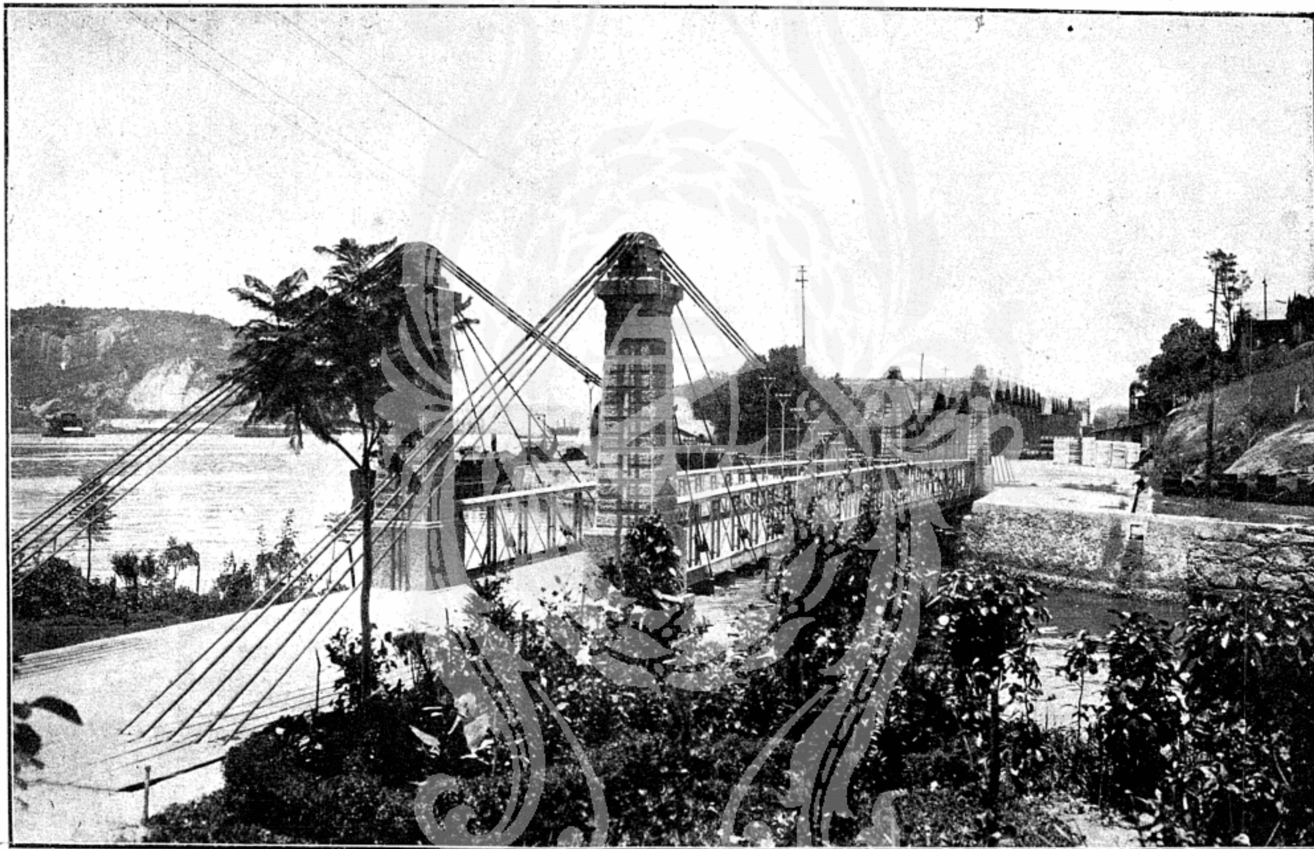
PONTE DE CABLES UNINDO A ILHA DO VIANNA E SANTA CRUZ, PROJECTADA PELO ENGENHEIRO FRANCIS M. ARNOLD E EXECUTADA, SOB A DIRECÇÃO DO COMPETENTE ENGENHEIRO JOSÉ LUIZ COELHO, VENDO-SE OS IMPORTANTES ESTALEIROS DE LAGE IRMÃOS, CREAÇÃO DO SAUDOSO INDUSTRIAL ANTONIO MARTINS LAGE.
